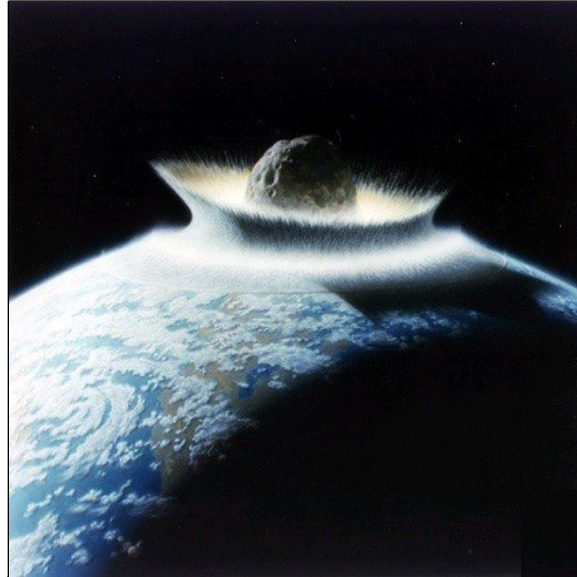
Simulación de un impacto de asteroide.
